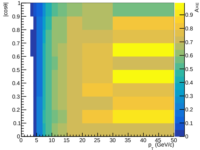
B \rightarrow D^*
