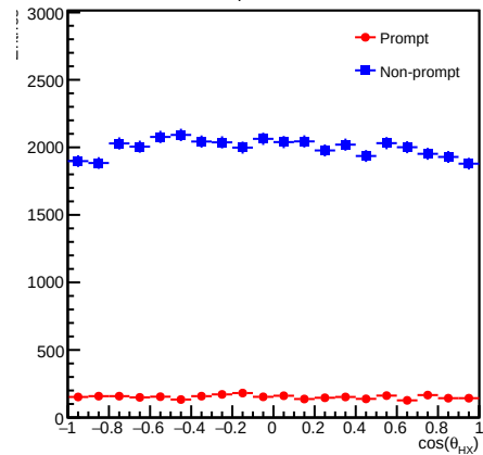
5 < p_T < 7 \text{ GeV/c}
