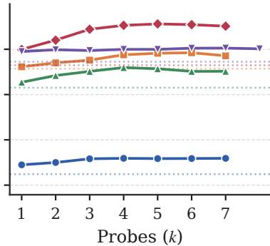
Llama-3.1-8B
