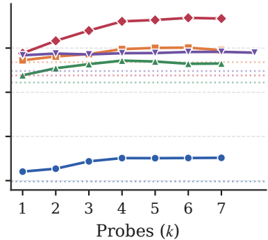
Mistral-7B
