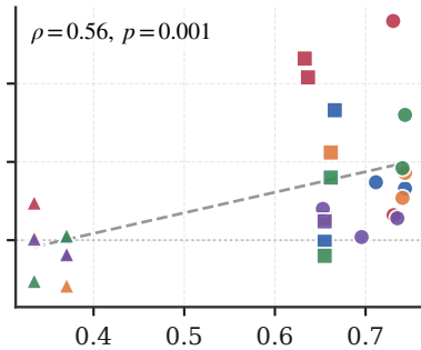
Mistral-7B
