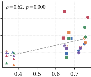
Llama-3.1-8B
