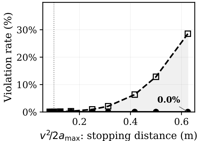
(d) Braking distance
