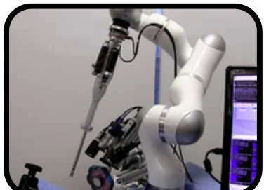
Kuka Med 14
