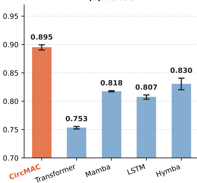
(b) AUROC
