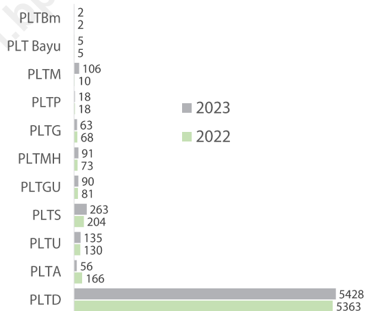
Gambar 10.3 Jumlah Unit Pembangkit Milik PLN di Indonesia Berdasarkan Sumber Energi
