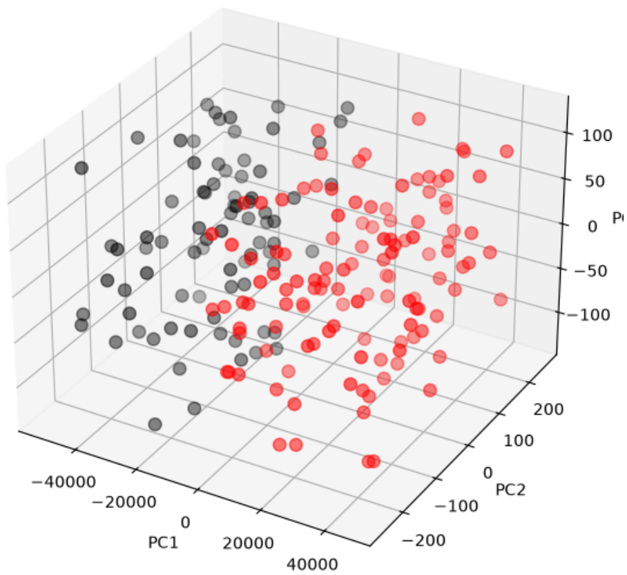
Hierarchical Clustering 3D PCA
