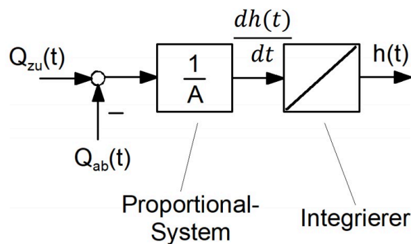
Figure 1: Blockschaltbild Füllstand
