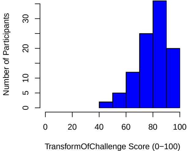
TransformOfChallenge Score
