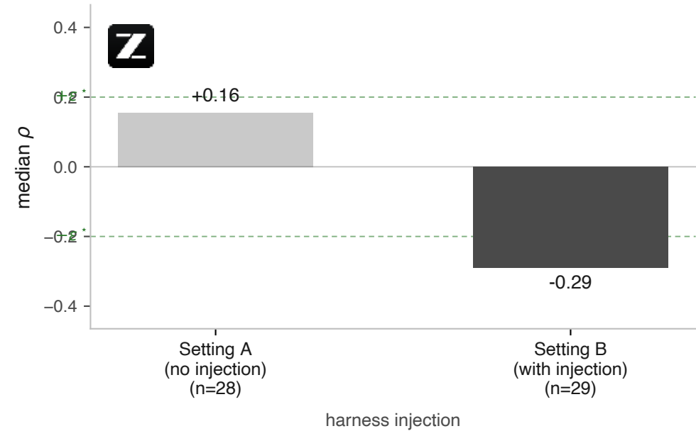
(d) Cross-vendor · GLM-5.2 ± date injection
