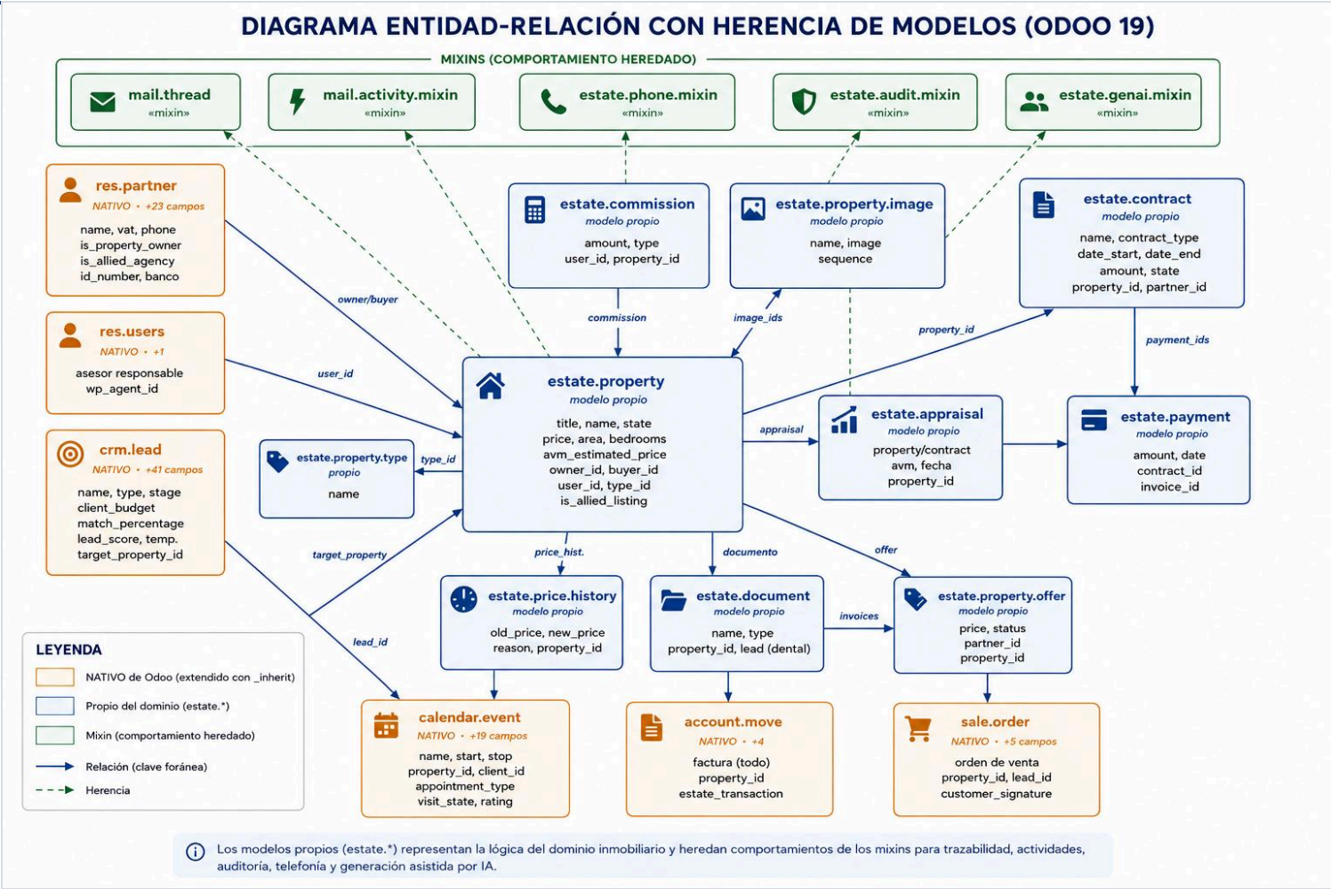
Figura 2 — Entidades núcleo y mixins reutilizables (Odoo 19)
