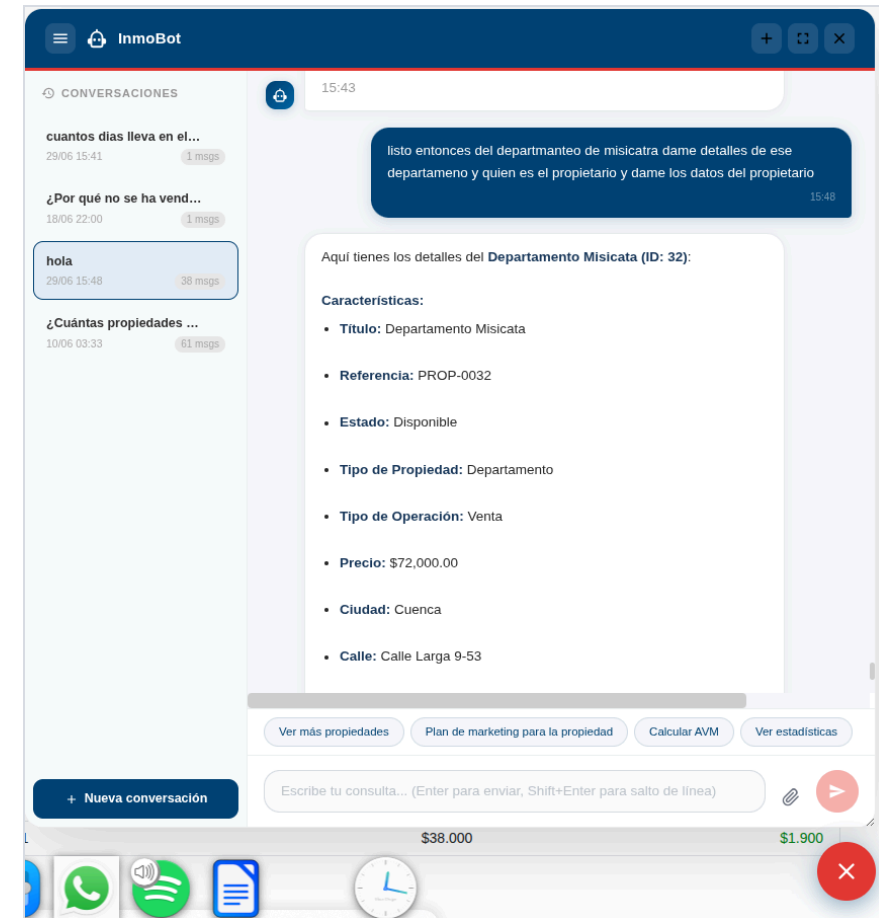
Figura 9 — Conversación real con el agente
