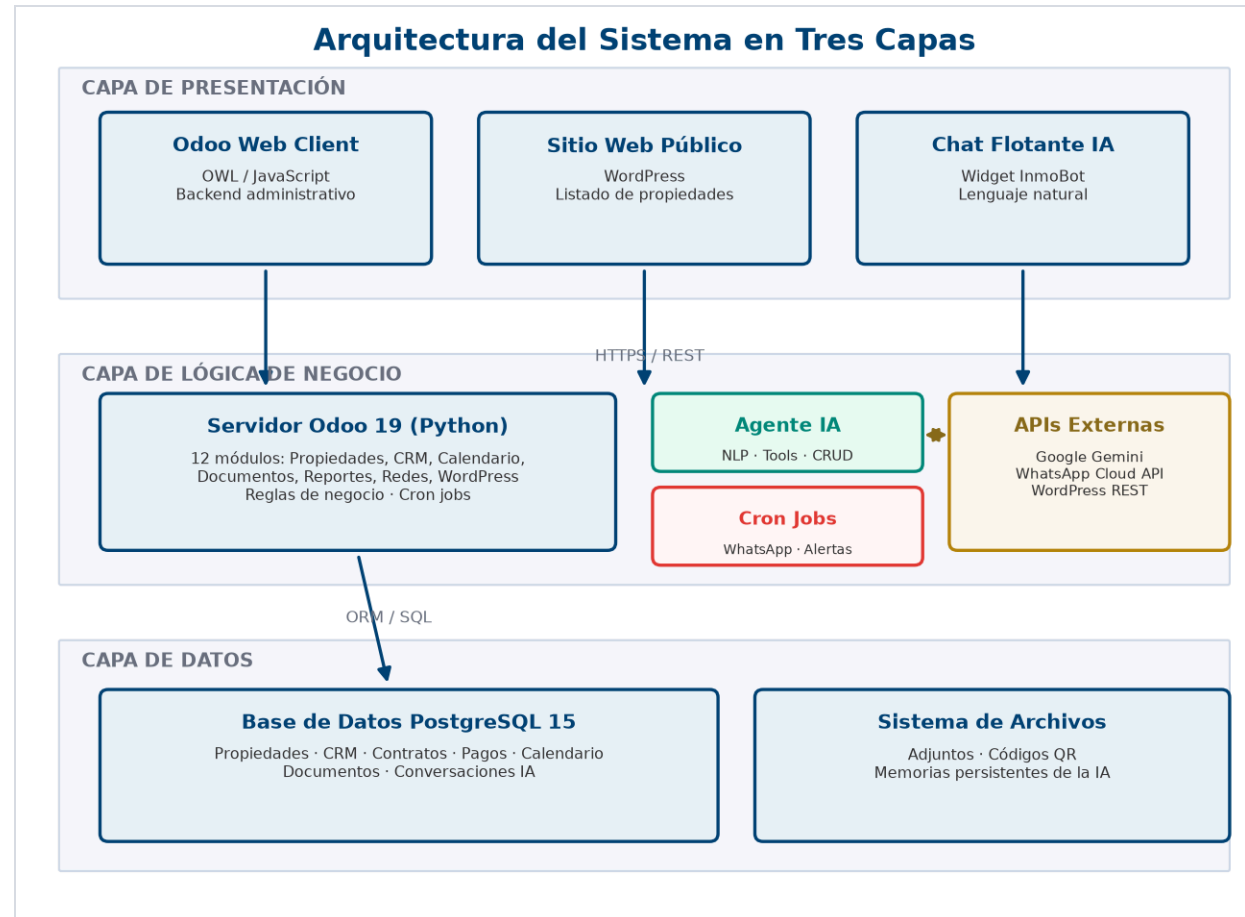
Figura 4 — Presentación · Lógica de negocio · Datos
