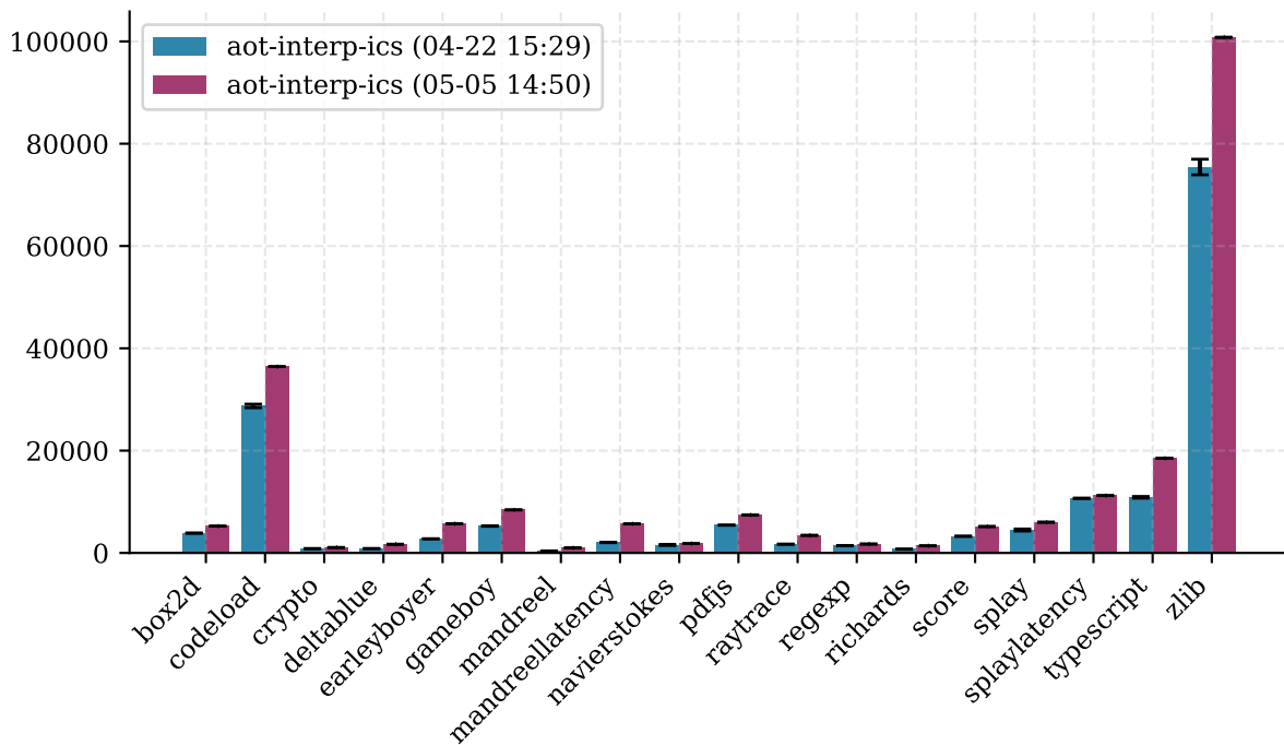
Octane Sub-benchmarks
