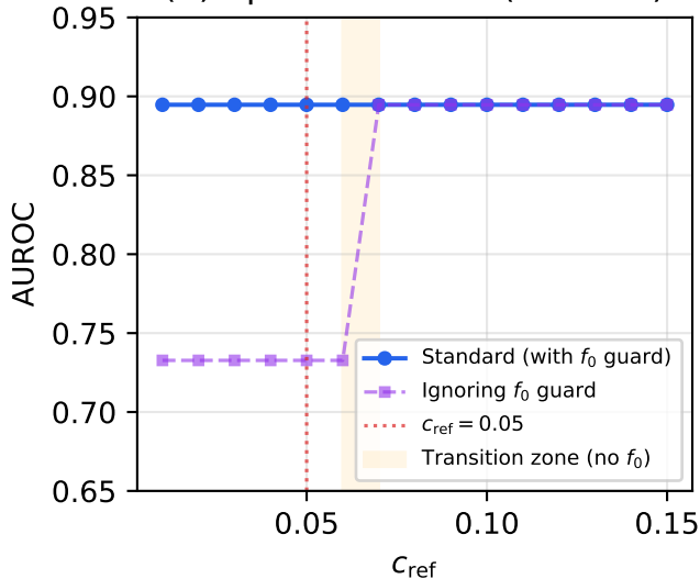
(b) SparseDOSSA2 ( N = 500 )
