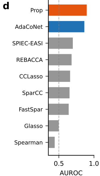
SparseDOSSA2 (N=500)
