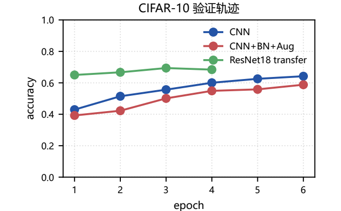
图 15: 不同模型的验证轨迹。训练轮数较少时，增强模型的收益可能滞后出现。
