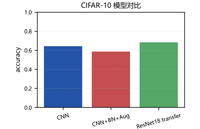
图 14: CIFAR-10 模型对比。迁移特征在小样本和短训练下具有明显效率优势。
