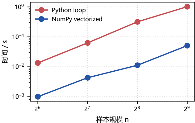
复杂度相同但常数差异巨大
