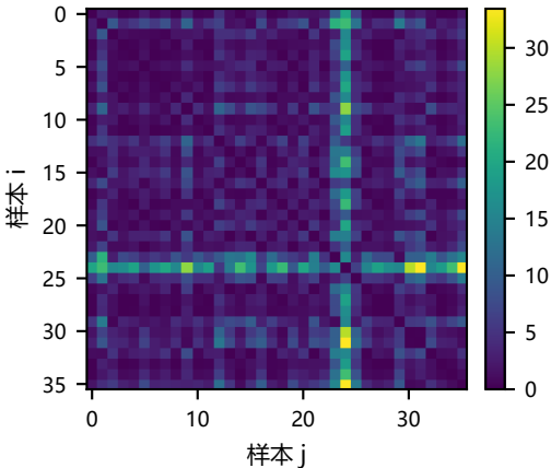
样本平方距离矩阵
