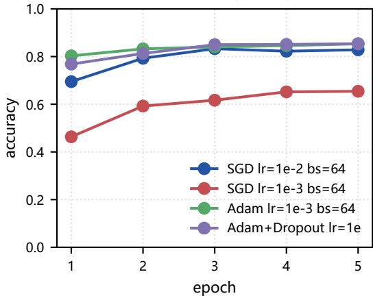
FashionMNIST 测试准确率
