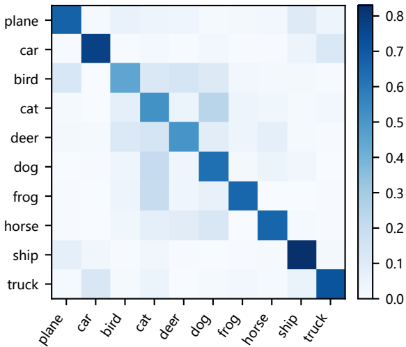
CIFAR-10 混淆矩阵
