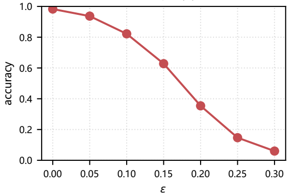
FGSM 攻击曲线
