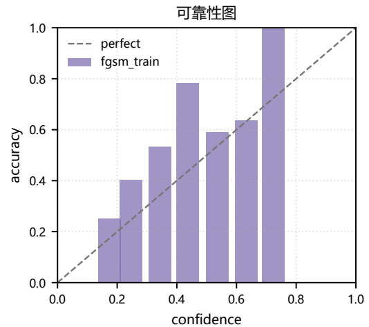
图 32: 可靠性图。对角线表示置信度与经验准确率完全一致。
