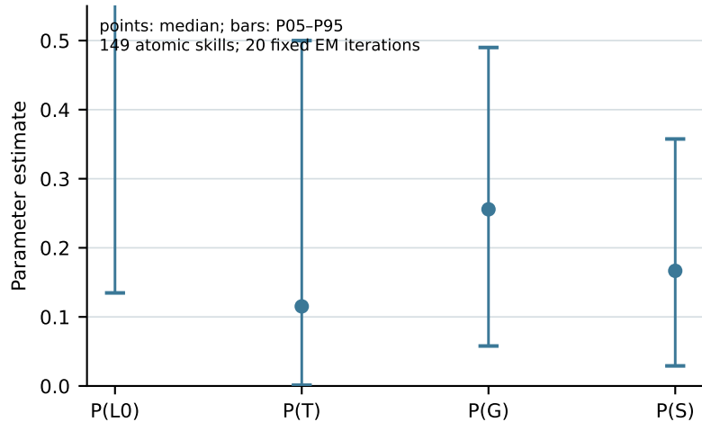
Across-skill BKT parameter summaries
