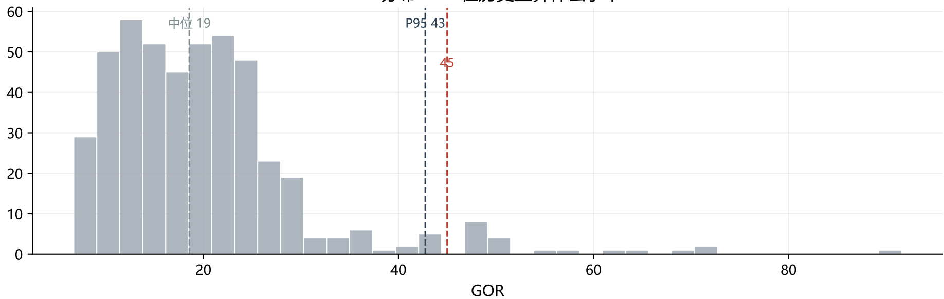
GOR 分布: 45 在历史里算什么水平?
