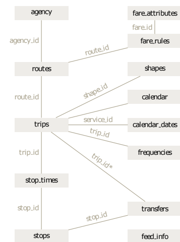
Abbildung 4: Aufbau der General Transit Feed Specification.
