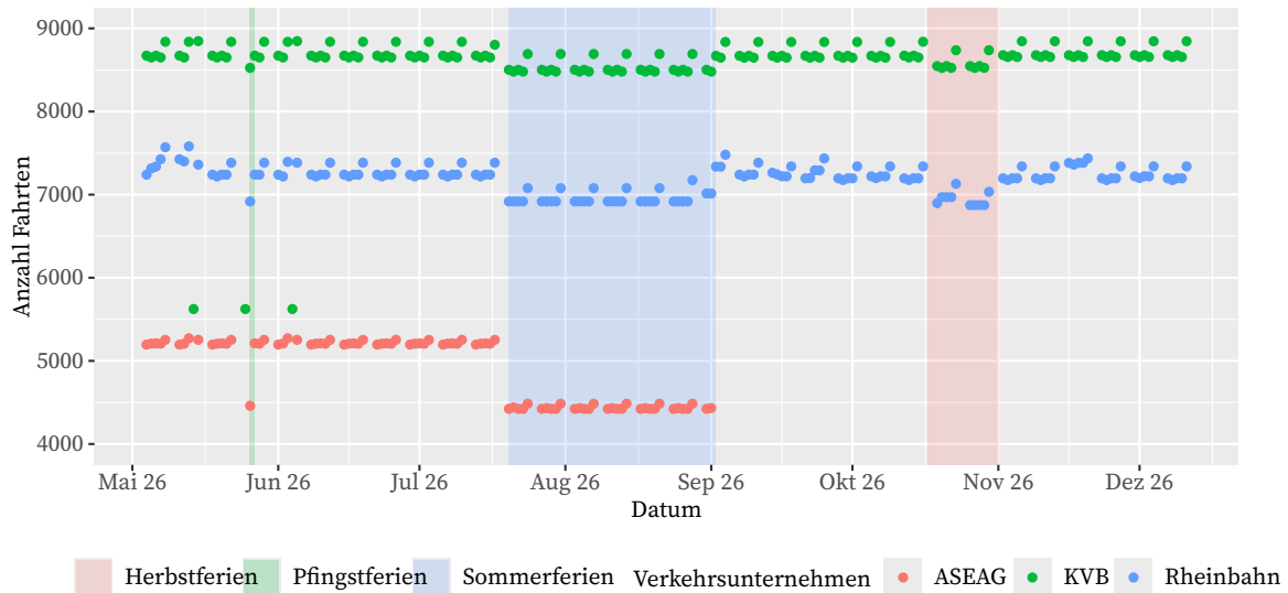
Abbildung 4: Fahrten (trips) je Wochentag der drei größten Verkehrsunternehmen nach Fahrten auf Grundlage des DELFI-GTFS vom 18.05.2026. Die Zahlen der Rheinbahn und ASEAG für die Feiertage in Mai und Juni liegen außerhalb der Skala.
