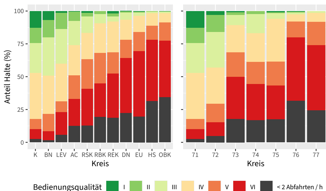
Abbildung 12: Anteil der Halte nach Bedienungsqualität (Median der Stunden), aggregiert nach Kreis bzw. regionalstatistischem Raumtyp (RegioSta7 (BMDV 2026))
