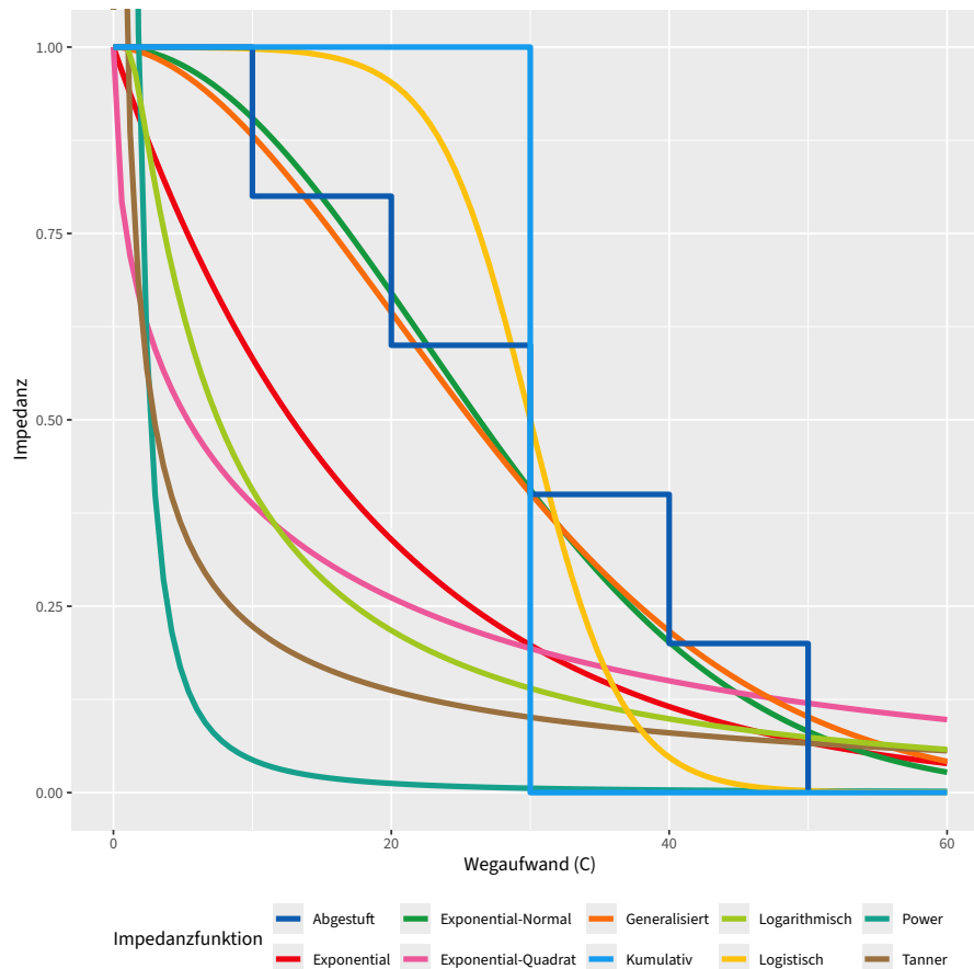
Abbildung 3: Verlauf verschiedener Impedanzfunktionen zur Verwendung mit der Hansen-Formel nach LEVINSON & KING (2020: 49), vgl. B2-22
