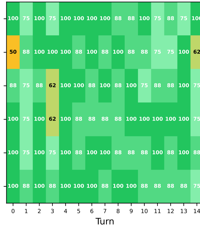
GLM-5.2
