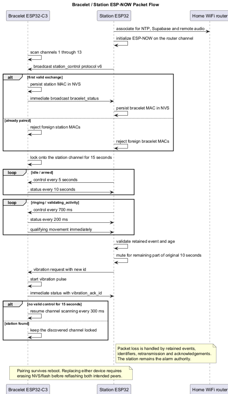
Diagramme : flux des paquets ESP-NOW
