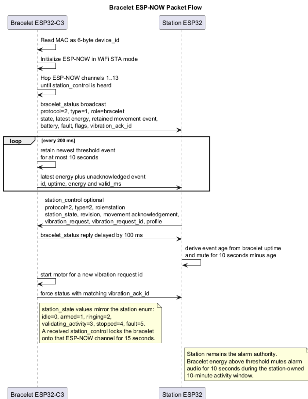
Diagramme : flux des paquets ESP-NOW
