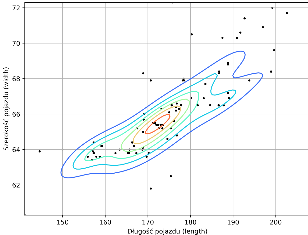
Dwuwymiarowa estymacja funkcji gęstości (KDE)
