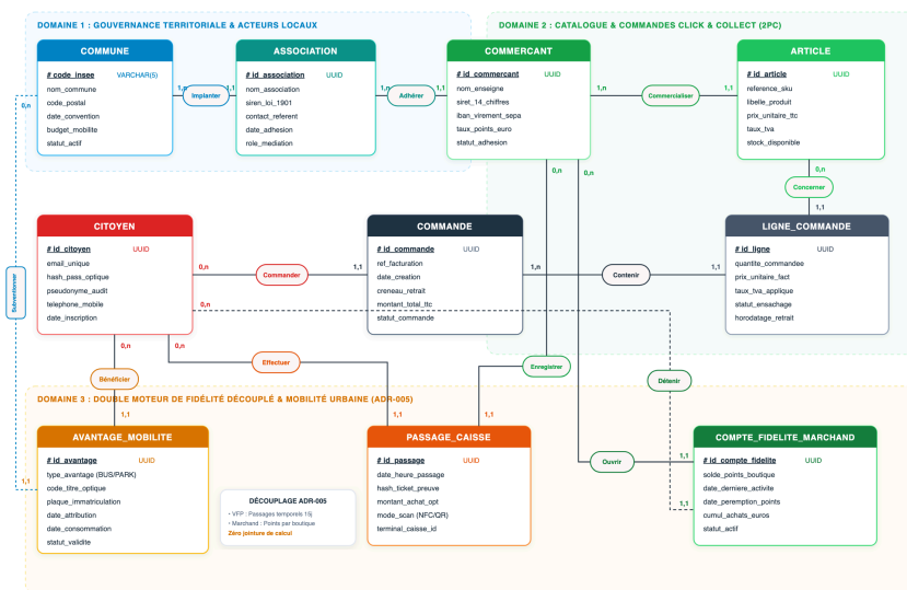
Figure 4.1 — Modèle Conceptuel de Données (MCD Merise) & Découplage des Moteurs de Fidélité (ADR-005)
