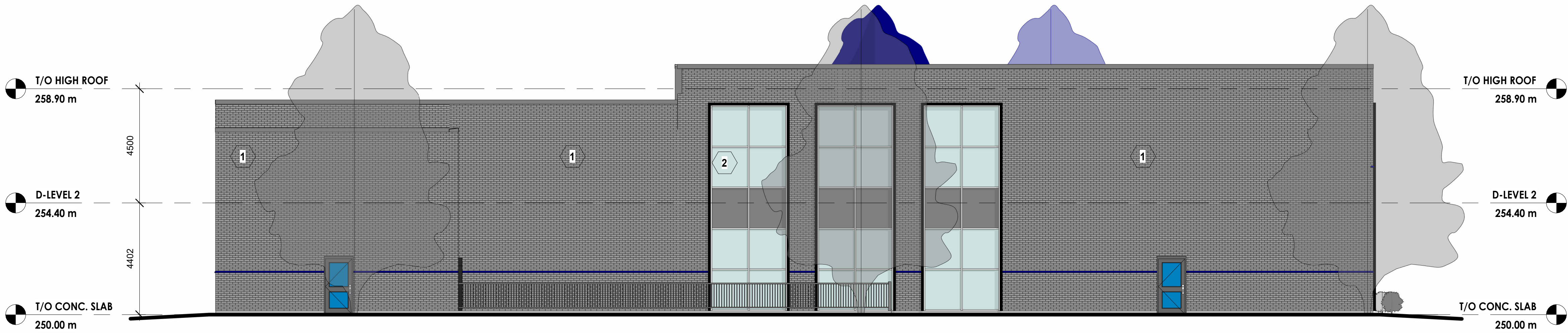
3 D-North 1 : 100
