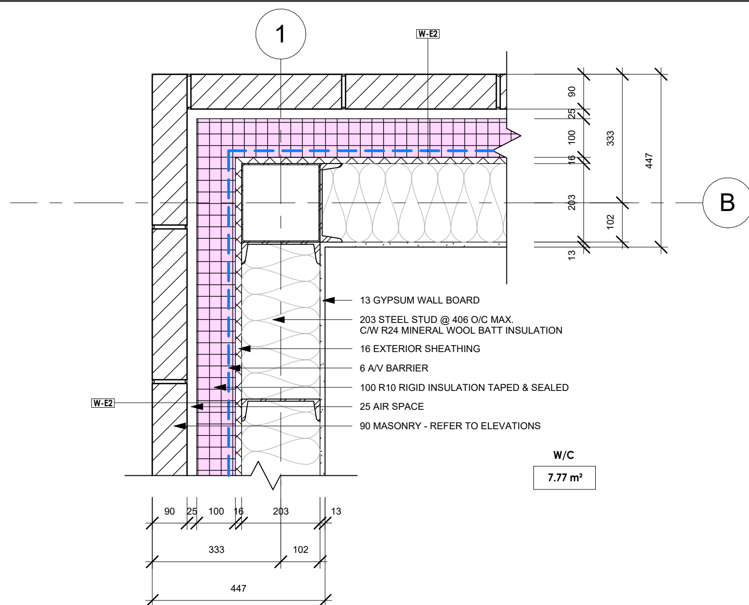
EXT. MASO. COR. PLAN DET. 1 : 10
