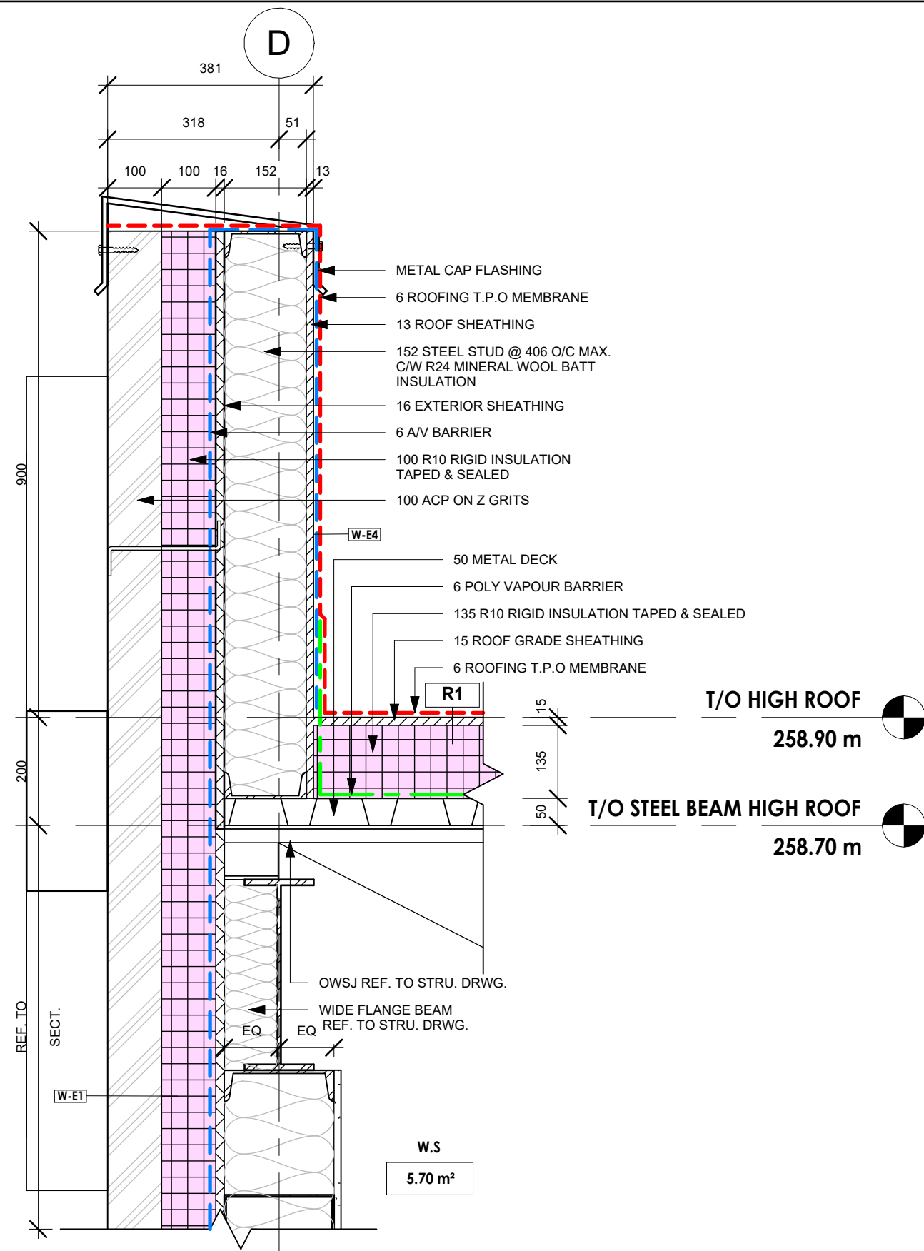
A.C.M PARA. SEC. DET. 1 : 10
