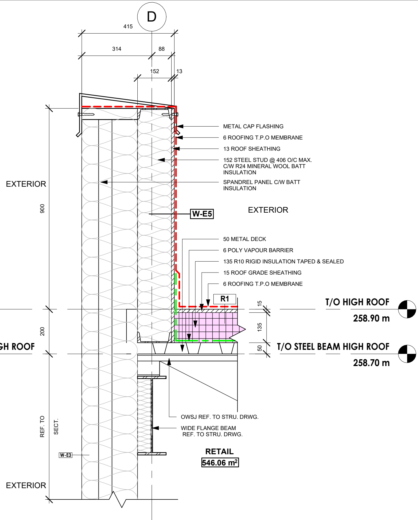
A.C.M PARA. SEC. DET. 1 : 10
