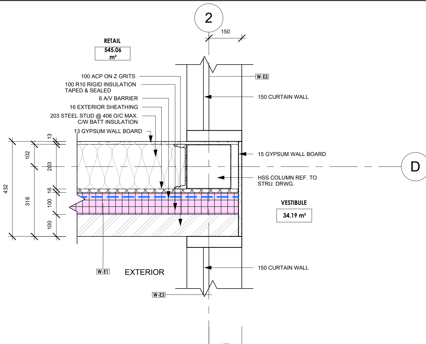
INT. COR. PLAN DET. 1 : 10
