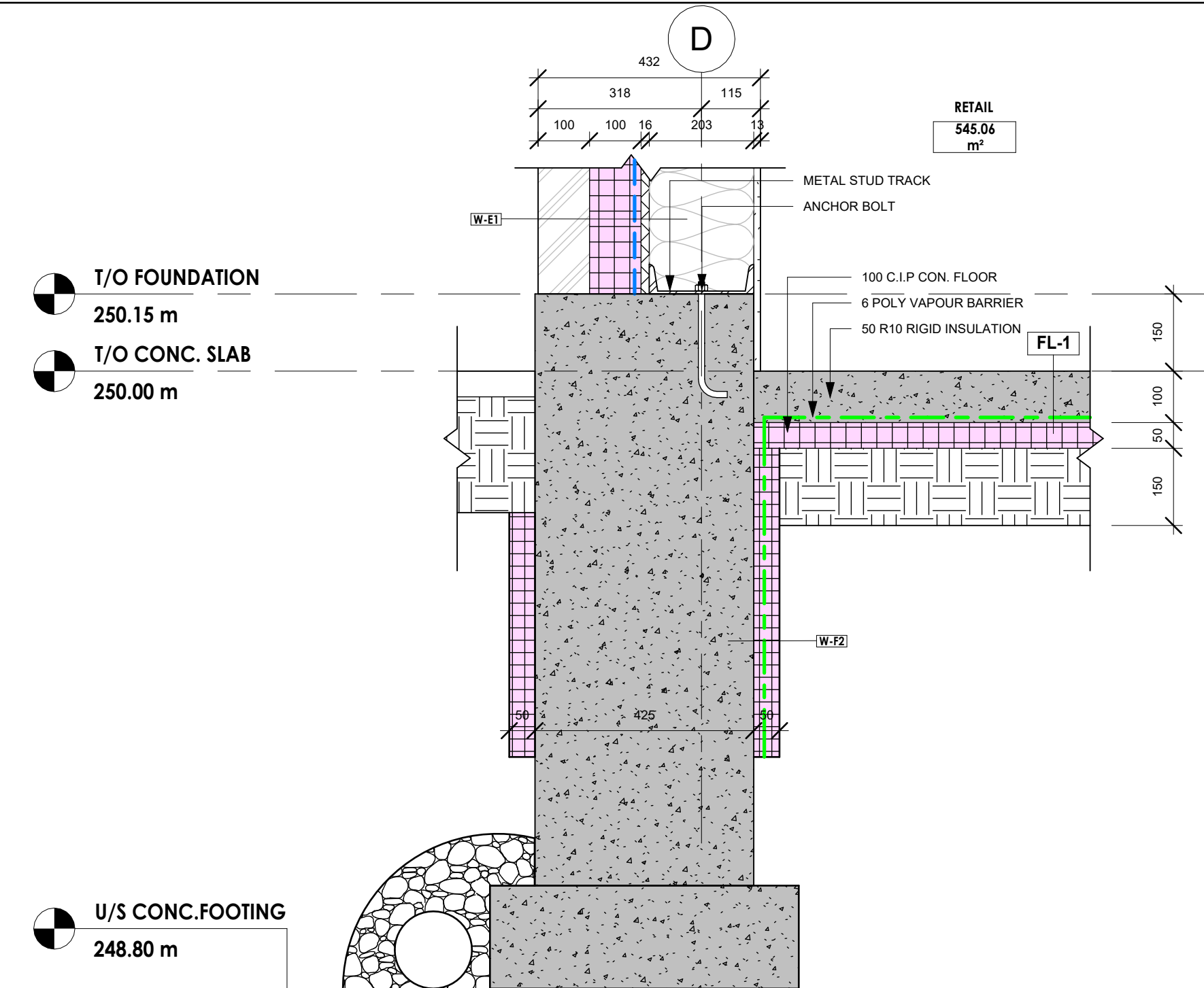
TYP. FOUND. DET. 1 : 10
