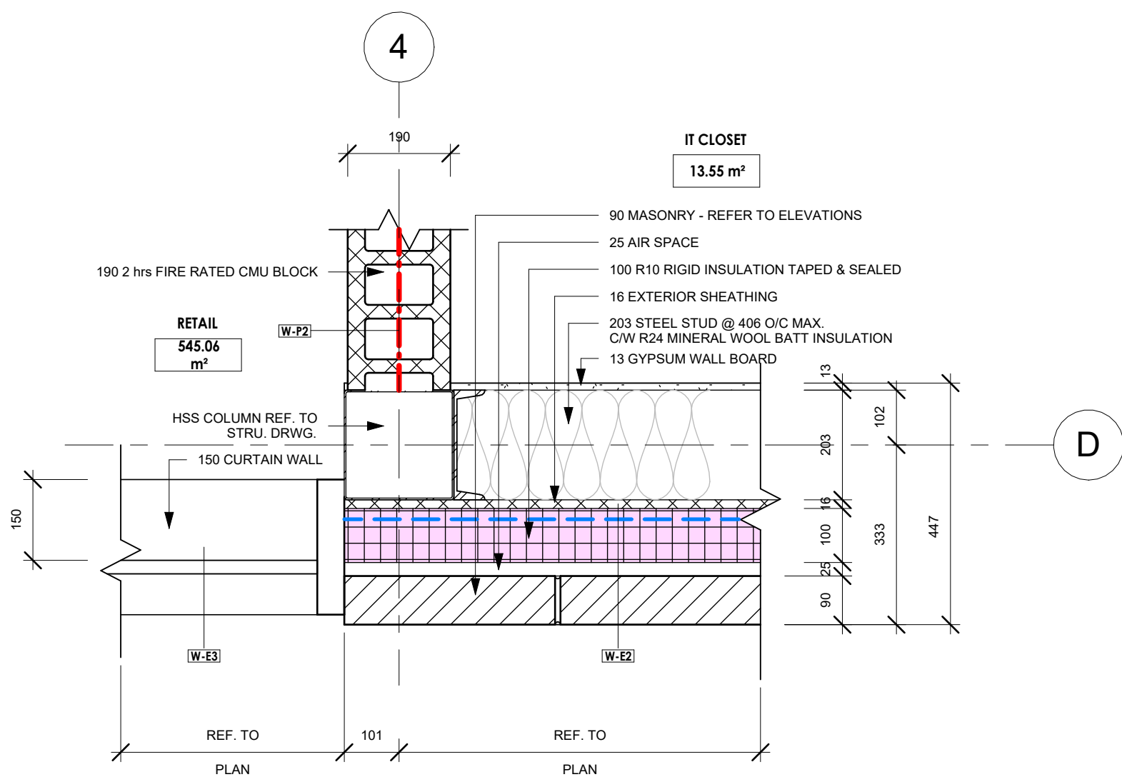
INT. COR. PLAN DET. 2 1 : 10
