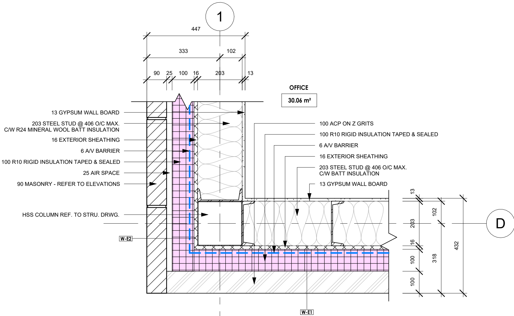
EXT. A.C.P COR. PLAN DET. 1 : 10
