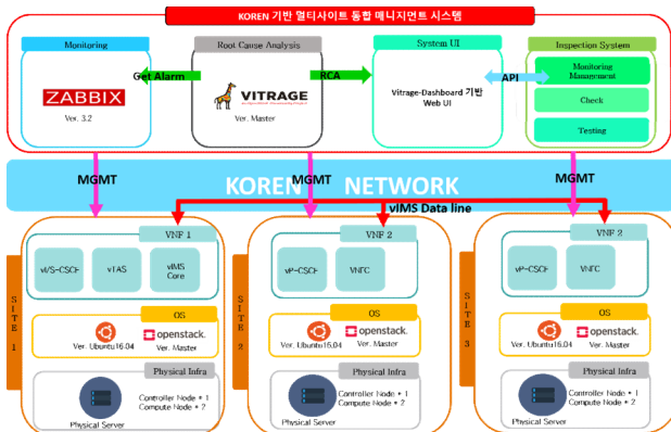
그림1. NFV 멀티사이트 환경 통합 관리 시스템
