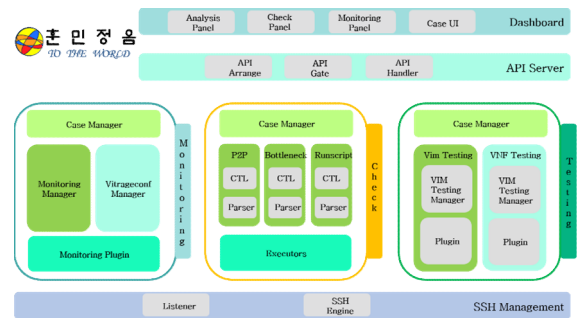
그림2. 세부 개발 내용
