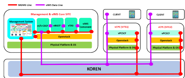
그림3. 멀티사이트 vIMS 컴포넌트 구성도
