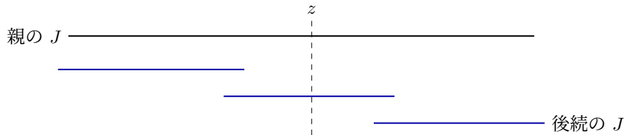
図 1: 後続による被覆の模式図. z を含む後続を選び, その後続でも同じ選択を繰り返す.
