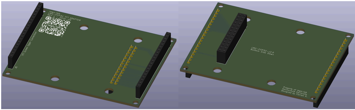
Abbildung 6: Vorderseite (rechts) und Rückseite (links) der Adapterplatine als 3D Rendering
