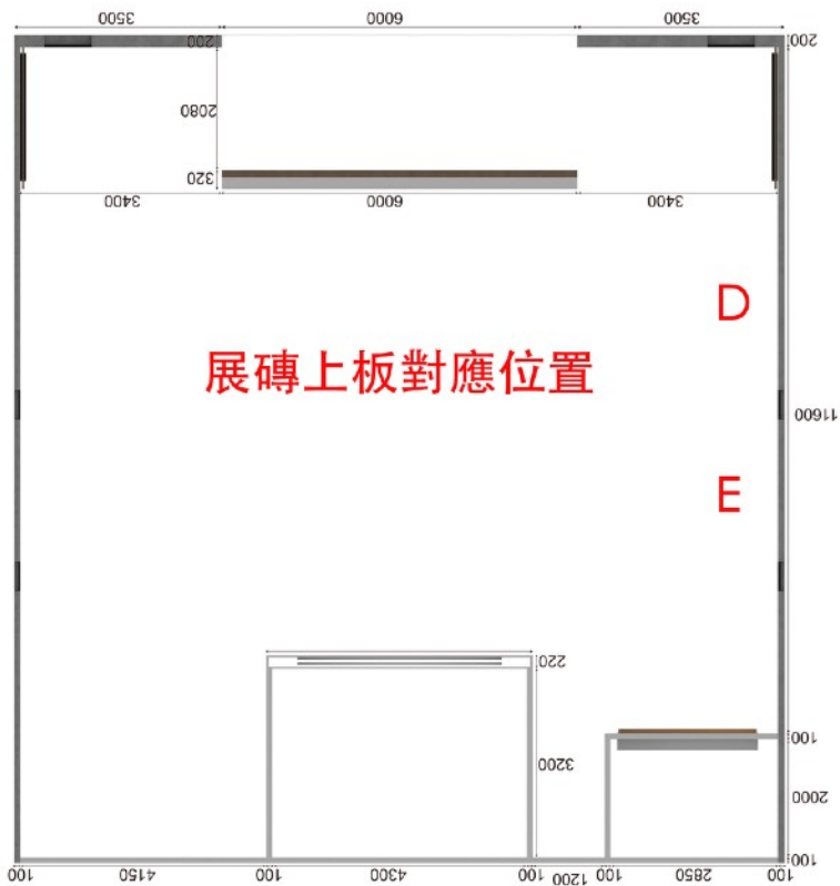
展場平面圖
