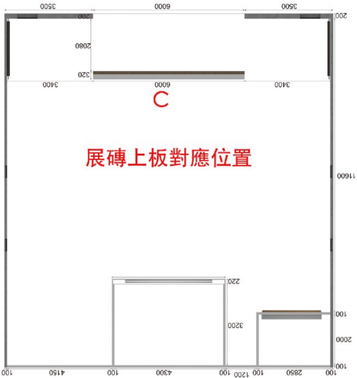
展場平面圖
