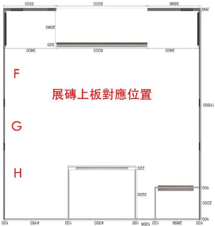
展場平面圖
