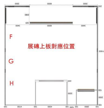
展場平面圖
