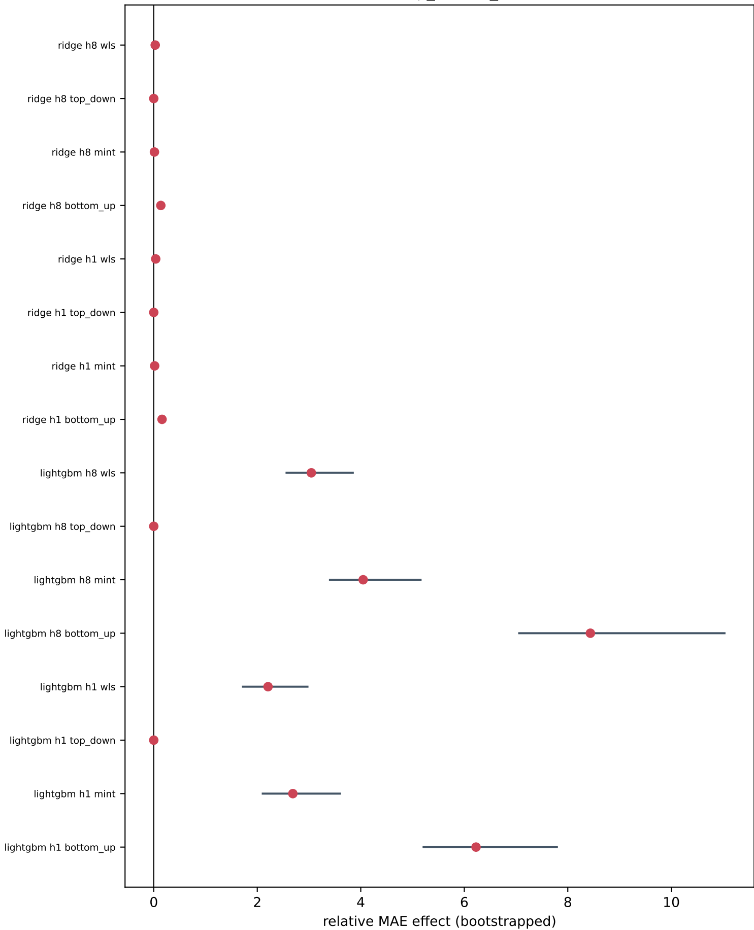
bootstrap_effects_disk
