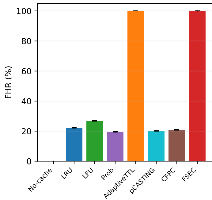
Comparaison des stratégies (cache = 100, SF7, batterie pleine)
