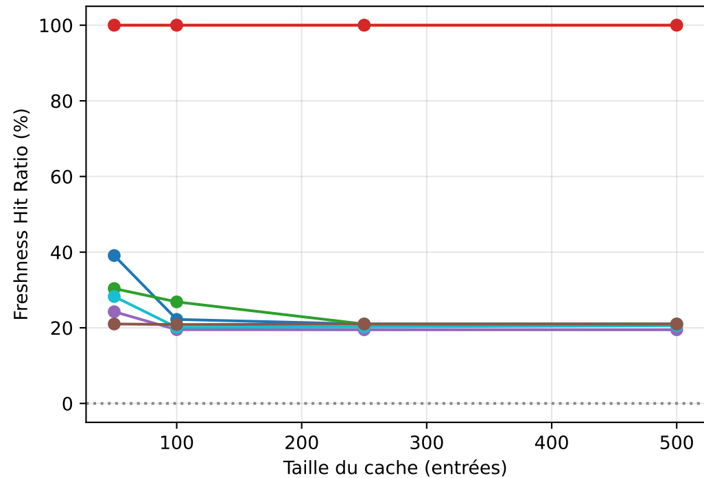
Performances en fonction de la taille du cache (IC 95 %)
