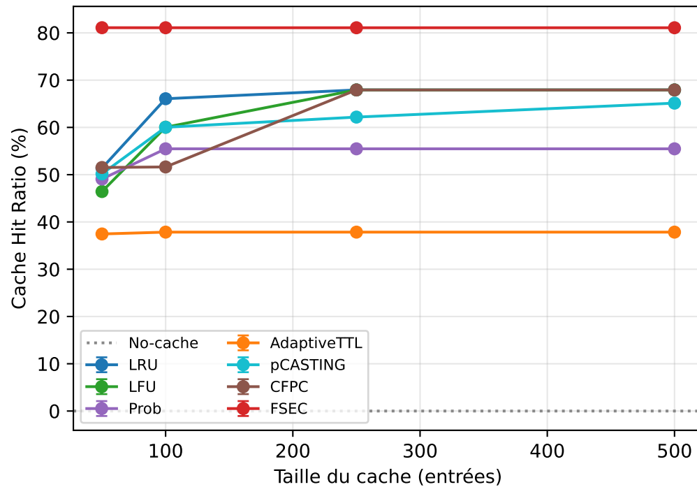
Performances en fonction de la taille du cache (IC 95 %)
