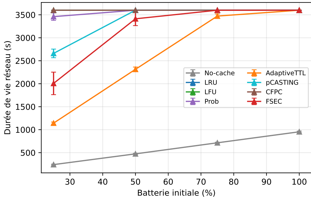
Effet du niveau de batterie initial (cache = 100, IC 95 %)
