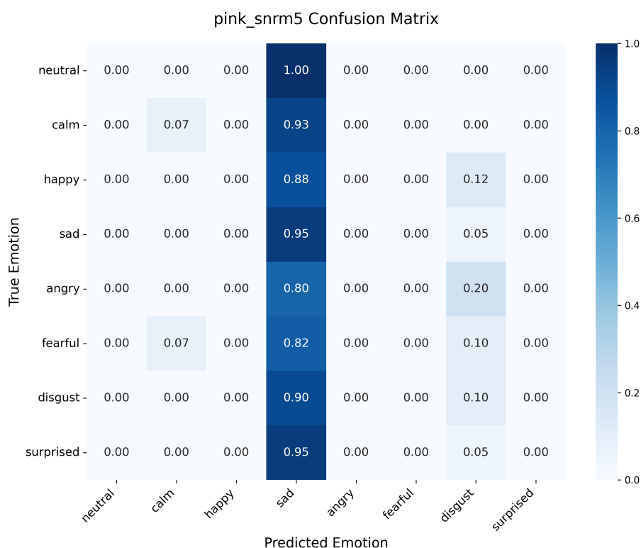
图 4-10 pink 噪声-5dB 条件下 CNN-Conformer 模型的混淆矩阵
