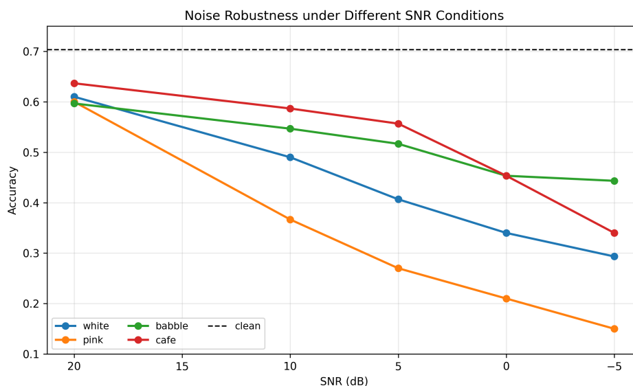
图 4-9 不同噪声强度下 CNN-Conformer 模型的 Accuracy 变化
