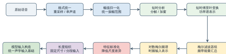
图 2-7 本文采用的信号处理流程
