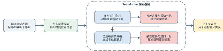
图 3-7 Transformer 编码器层的基本信息流动
