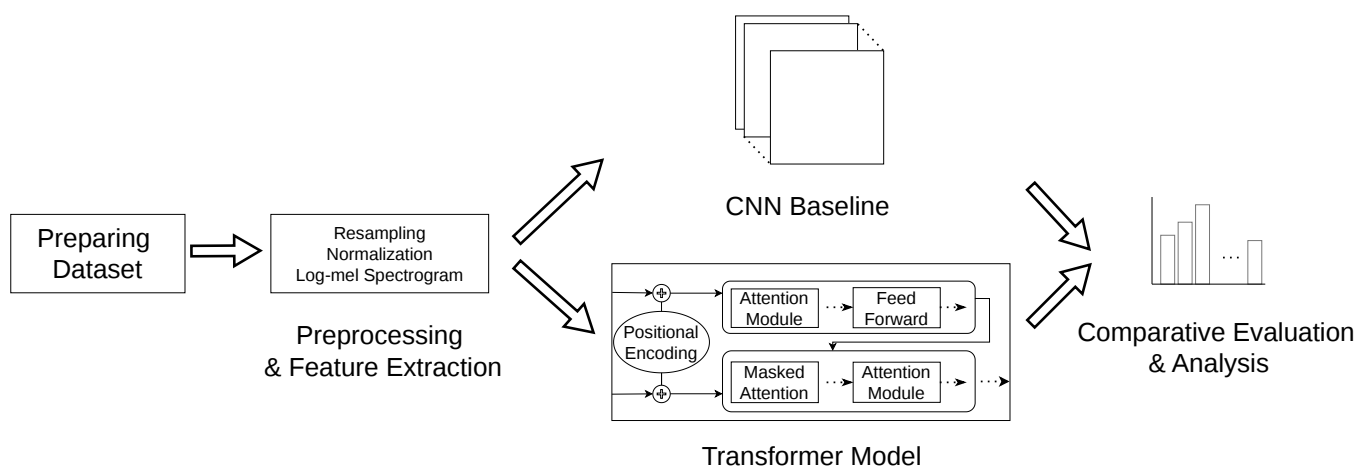
图 1-3 研究流程图：涵盖数据预处理、卷积神经网络模型与 Transformer 并行对比及结果分析
