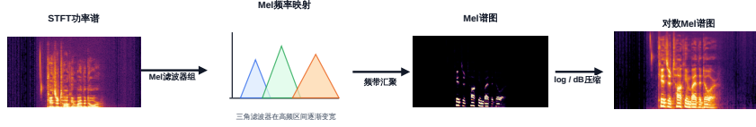
图 2-4 梅尔谱图与对数梅尔谱图的生成关系及动态范围差异
