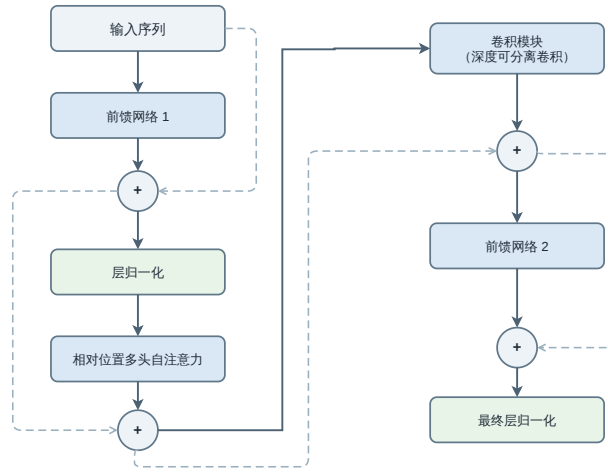
图 4-7 Conformer 编码块结构
