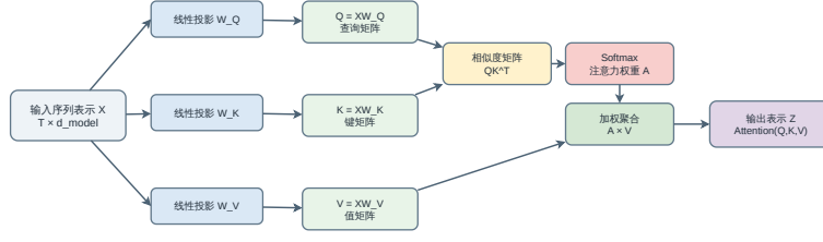
图 3-5 缩放点积注意力中的查询、键、值计算流程
