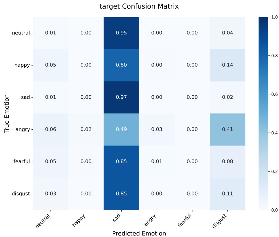
图 4-9 CREMA-D 目标语料上的混淆矩阵
