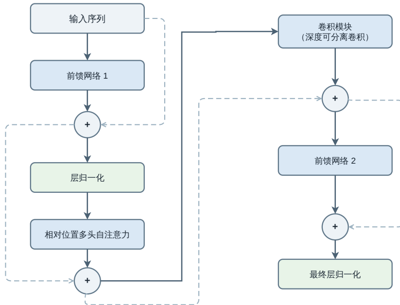
图 4-5 Conformer 编码块结构
