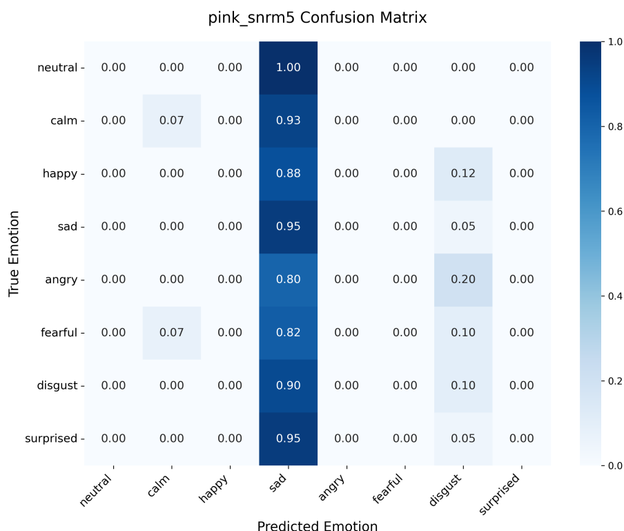
图 4-7 pink 噪声-5dB 条件下 CNN-Conformer 模型的混淆矩阵
