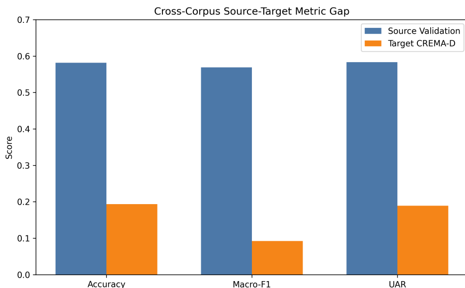
图 4-8 跨语料库实验中源验证集与目标语料的指标差距
