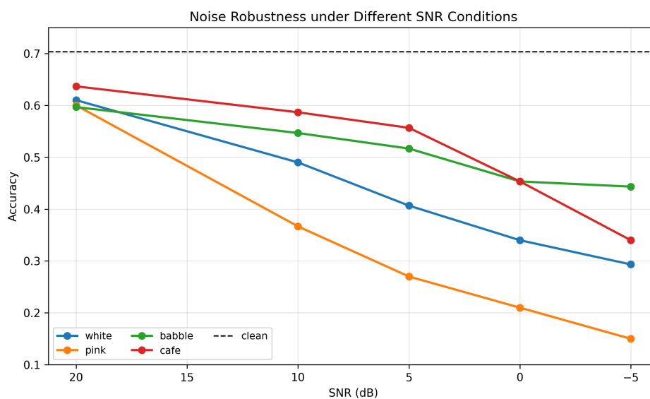
图 4-6 不同噪声强度下 CNN-Conformer 模型的 Accuracy 变化
