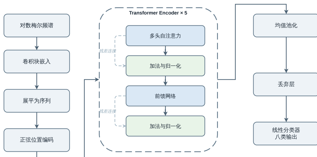
图 4-2 纯 Transformer 模型结构
