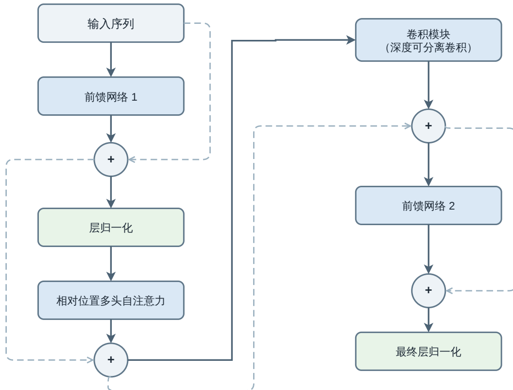
图 4-7 Conformer 编码块结构
