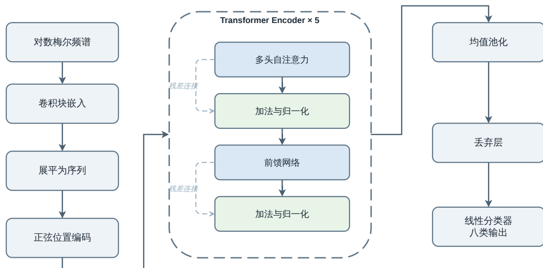
图 4-2 纯 Transformer 模型结构
